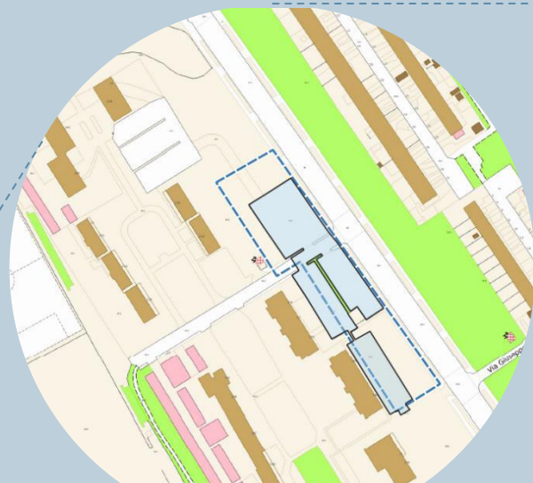
Disconnessione della rete del parcheggio di via della Repubblica mediante realizzazione di trincee drenanti e pozzi di infiltrazione
